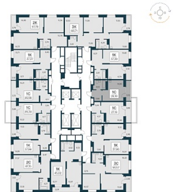
ПЛАН 12-23 ЭТАЖА
