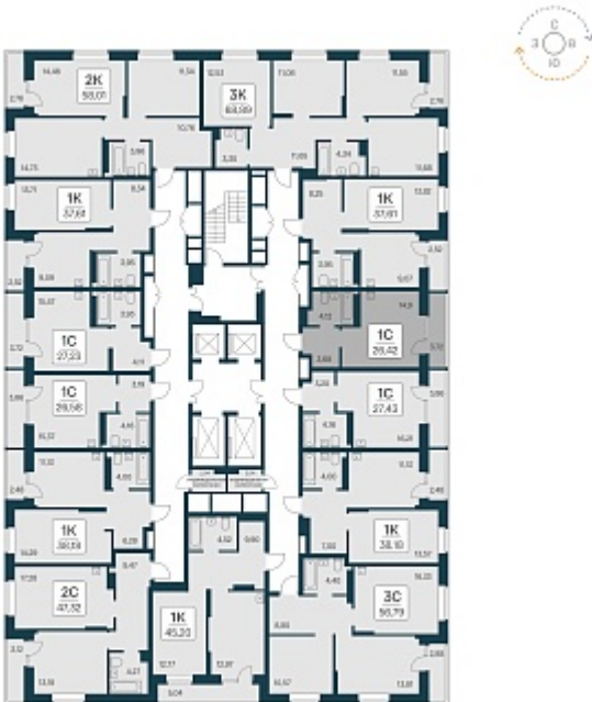
ПЛАН 2-11 ЭТАЖА
