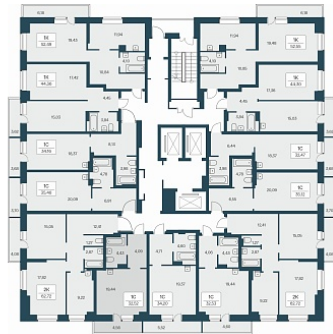
ПЛАН 10-27 ЭТАЖА
