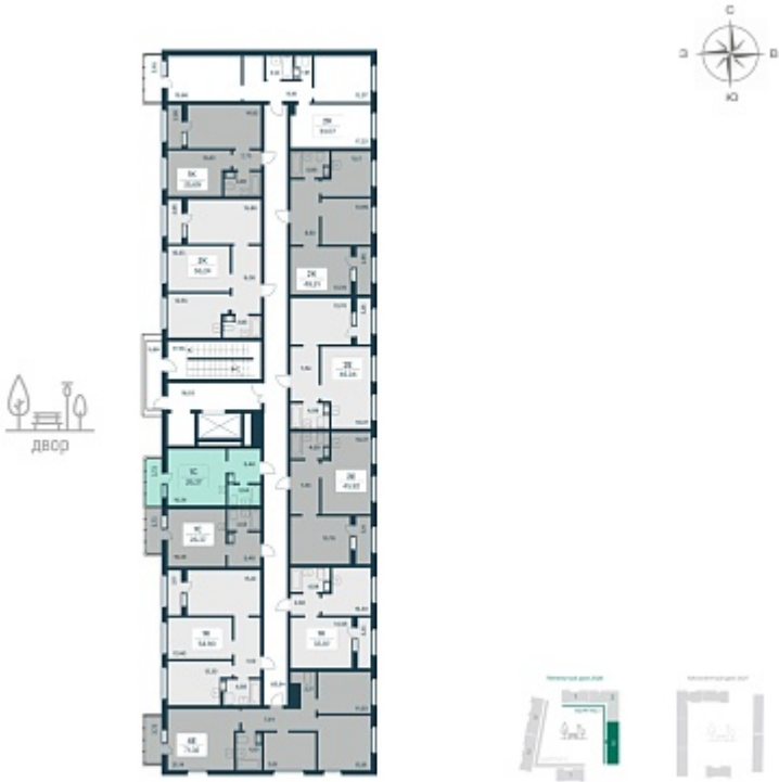
План этажа
