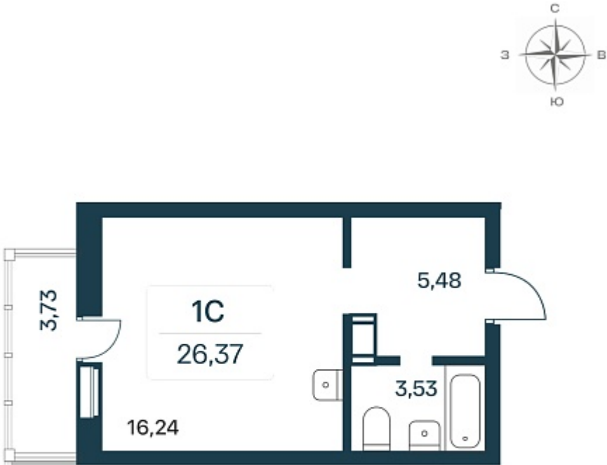
Планировка квартиры
